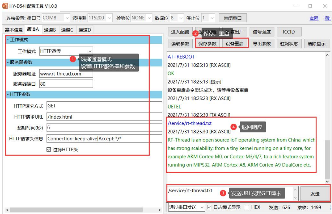
图 10 HTTP GET 请求
