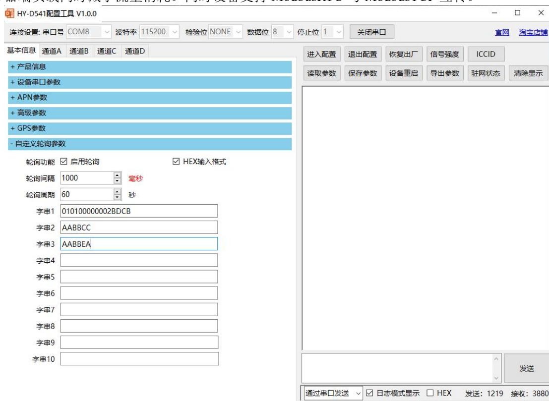
图 13 Modbus 轮询功能
