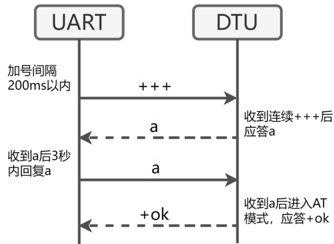
图 6 切换 AT 指令模式时序
