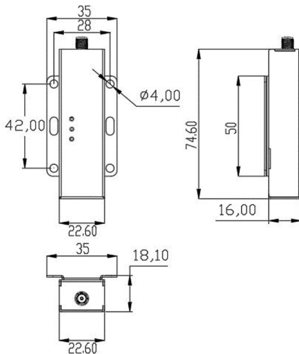
图 3 尺寸图 单位: mm
