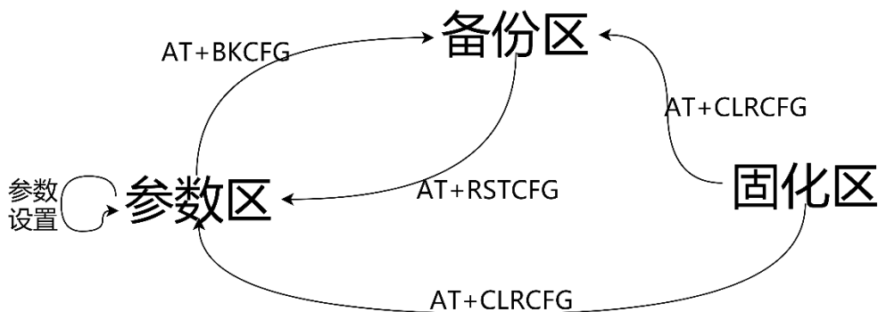
图 12 参数转换
