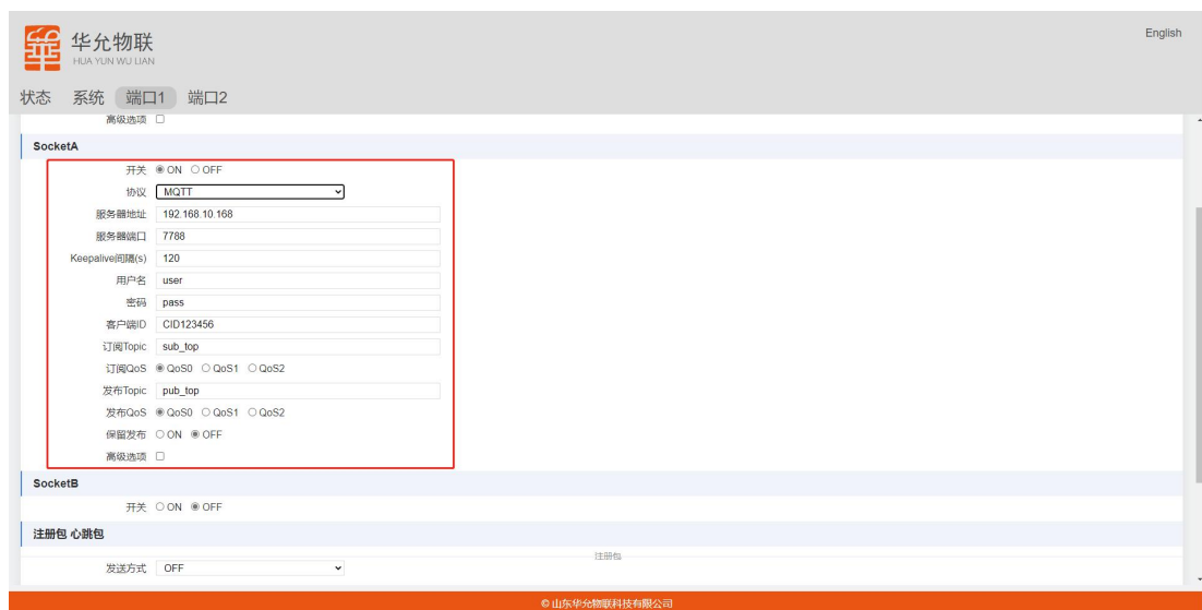
图 8 MQTT 参数设置
