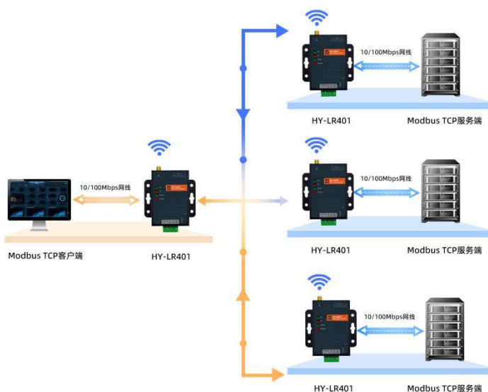
图-8 广播模式通信过程
