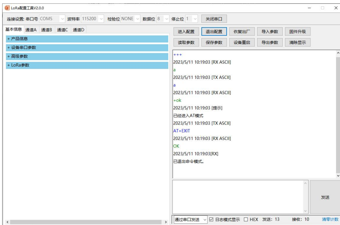
图-6 进入/退出配置模式
