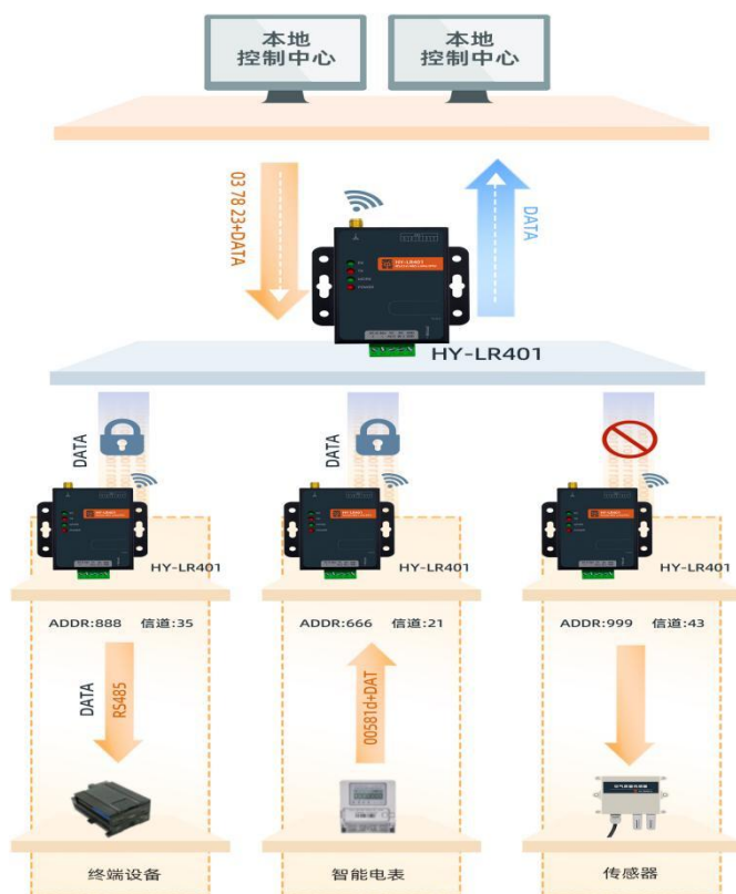
图-10 定点模式通信过程
