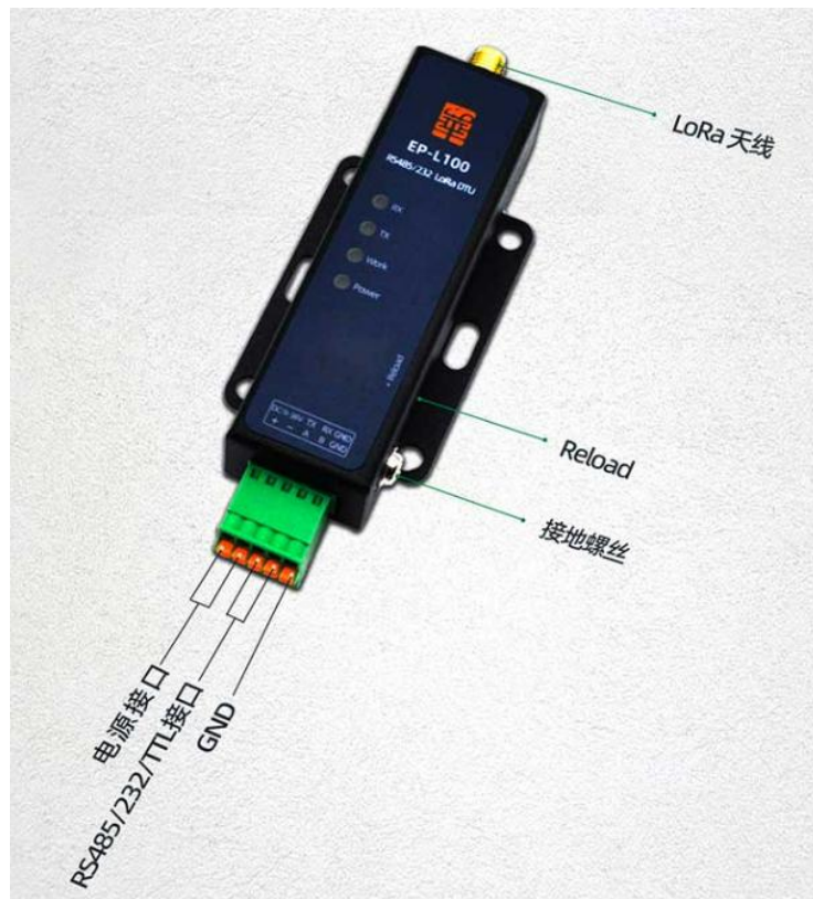
图-2 硬件接口
