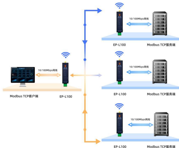
图-8 广播模式通信过程
