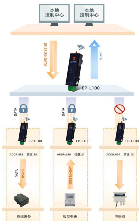
图-10 定点模式通信过程
