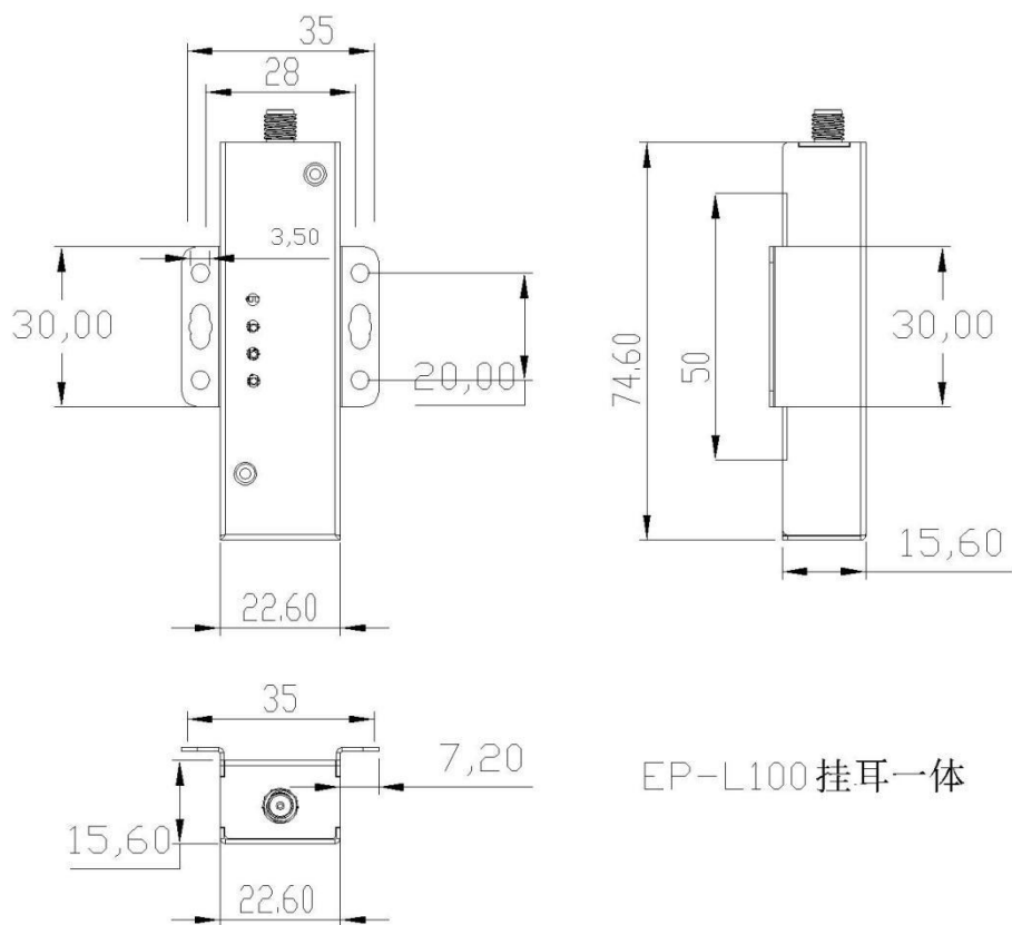
图-3 产品尺寸
